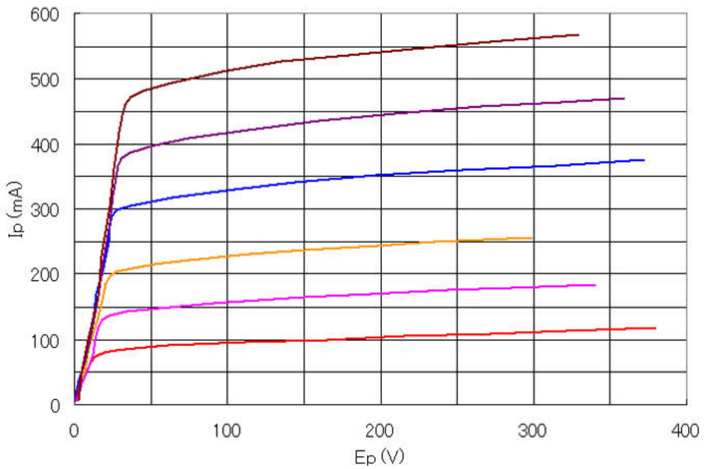
6GE5 Ep-Ip Curve Eg=0V
