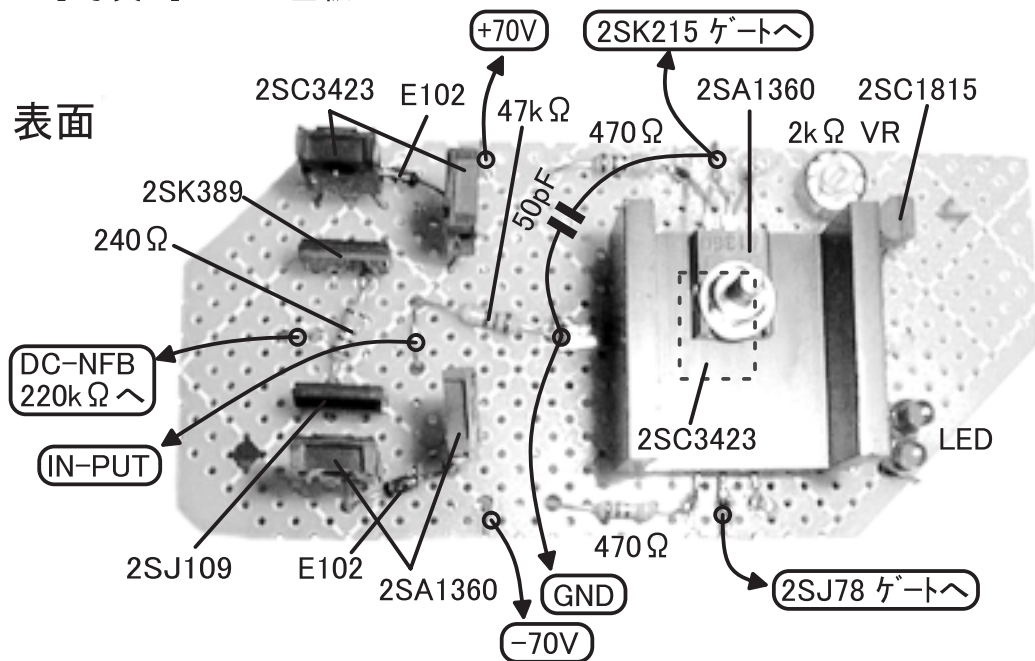
[ 写真 2 ] アンプ基板
