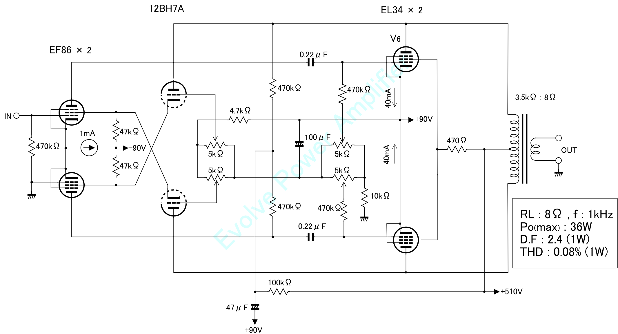
[ 図5 ] 超3結VXの実験回路
