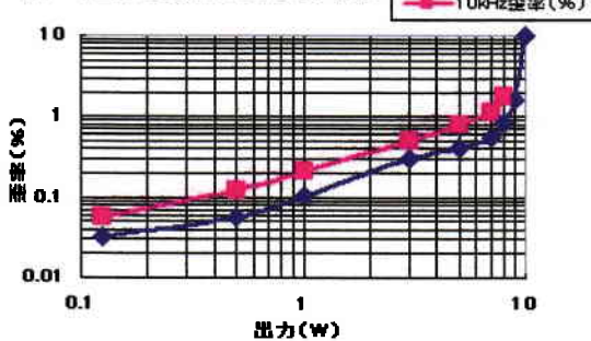
ムラード位相反転6V6pp歪率特性
