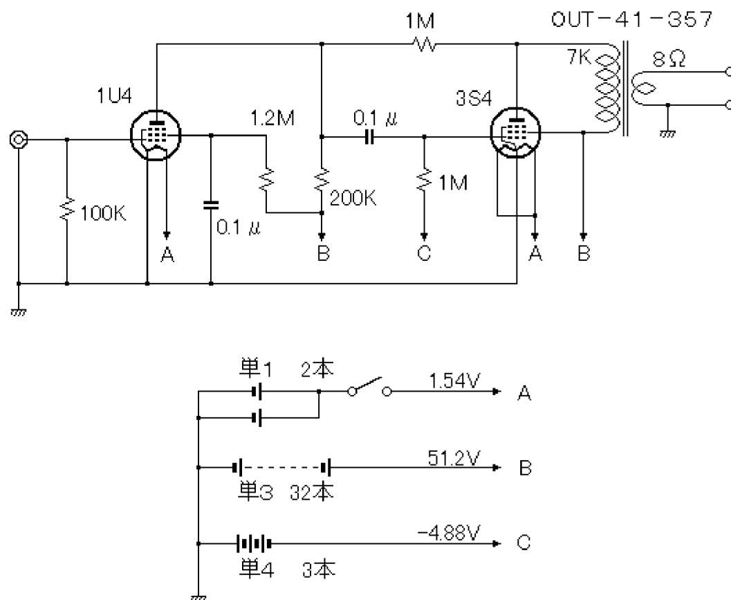
回路図
