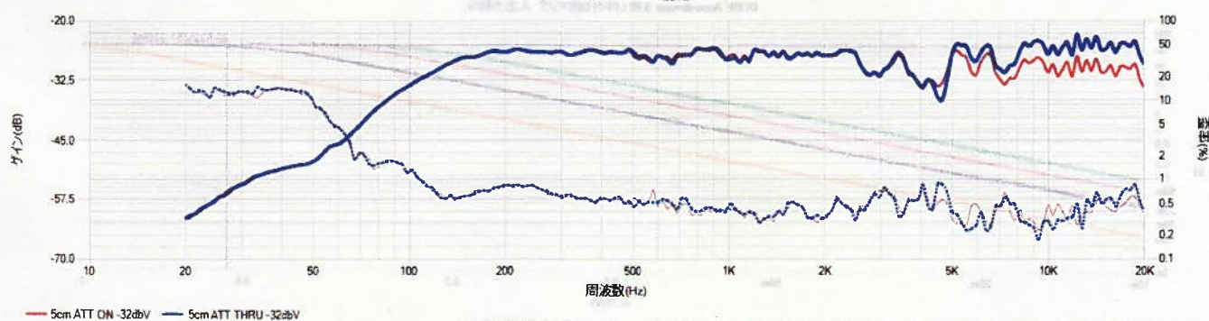
S-X33C ATT ON/OFF変化
