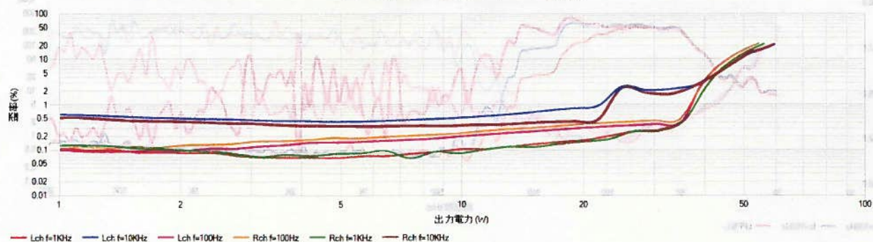
BOSE Acoustimass 5用 LPF付D級アンプ 出力対歪率特性
