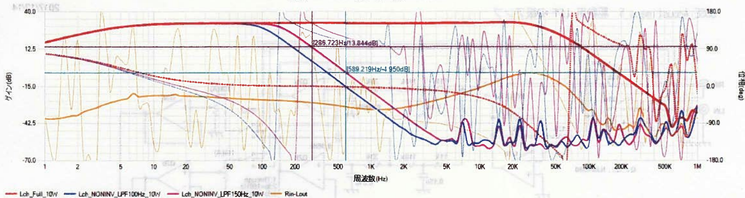
BOSE Acoustimass 5 用 LPF付D級アンプ 周波数特性
