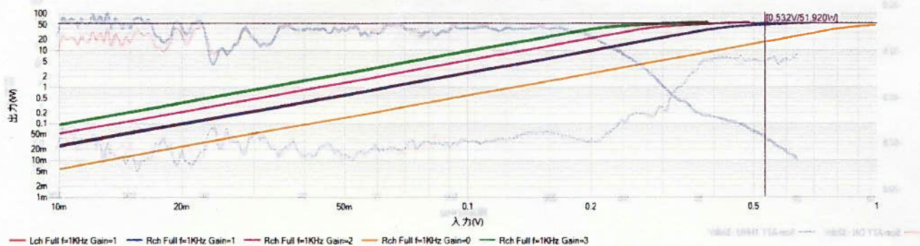
BOSE Acoustimass 5用 LPF付D級アンプ 入出力特性
