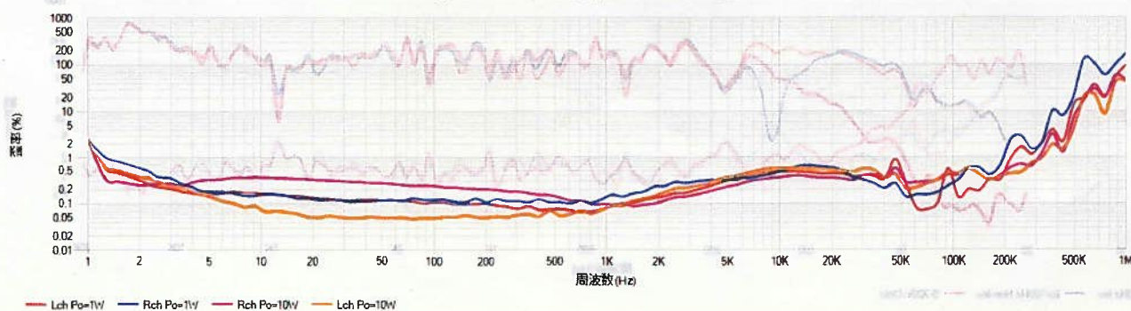
BOSE Acoustimass 5用 LPF付D級アンプ 周波数対歪率特性
