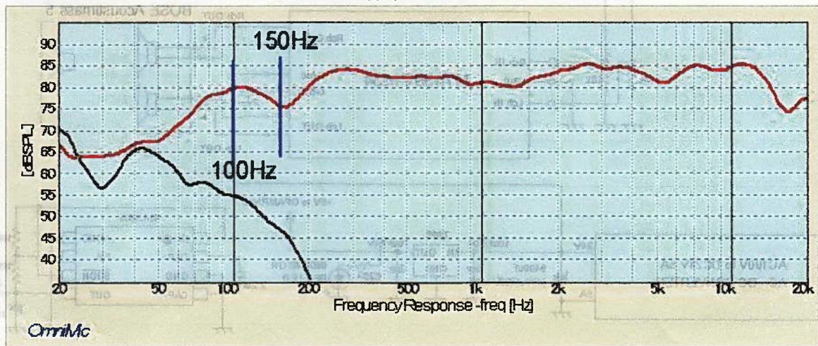
S-X33C ATT ON/OFF変化
