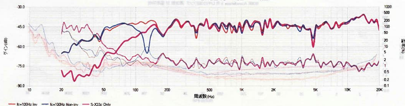
Pioneer S-X33C + Bose Acoustimass 5 合成音圧特性 Mic位置 S-X33c 軸上50cm
